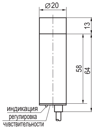
Габаритный чертёж
